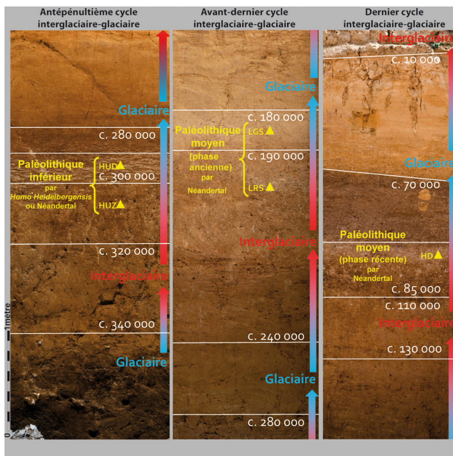
FIGURE 7 – Les différentes couches au nord de la Seine jusque 300 000 ans.
