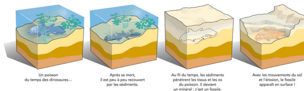
FIGURE 6 – Le processus de fossilisation.
