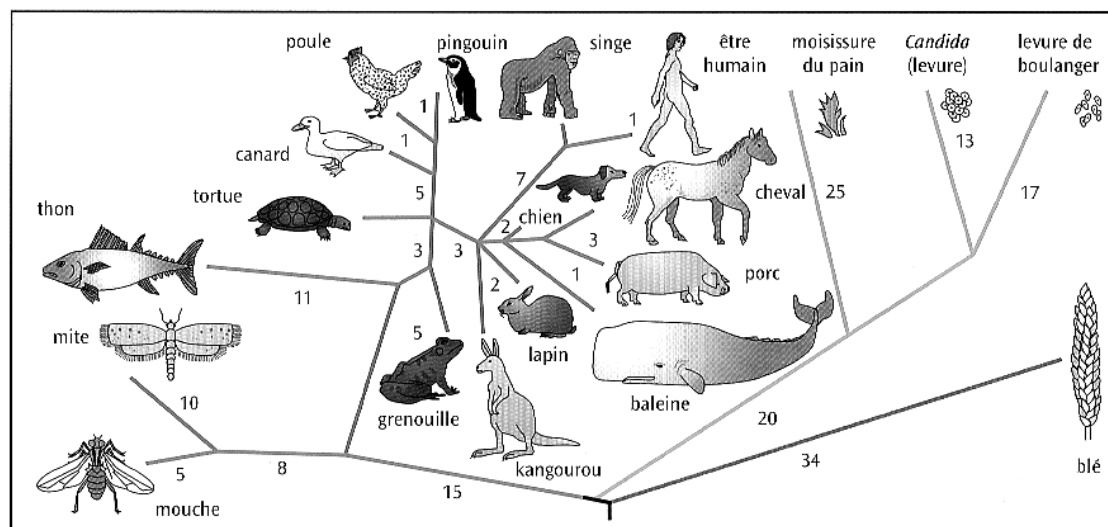
FIGURE 17 – L'évolution selon les modifications d'une protéine (le cytochrome C).
