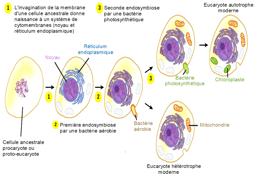
FIGURE 12 – L'endosymbiose des mitochondries et des chloroplastes.
