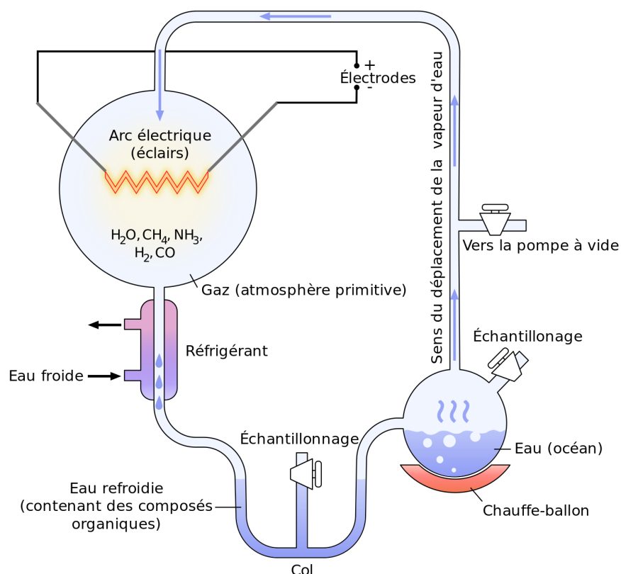
FIGURE 10 – L'expérience de Miller.
