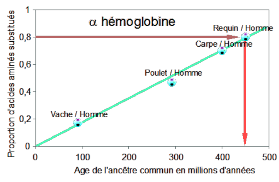
FIGURE 8 – Horloge moléculaire de l'hémoglobine des différents vertébrés.
