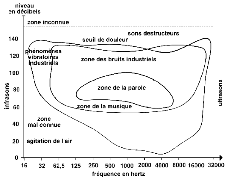
FIGURE 9 – Rapport entre décibels et fréquence.
