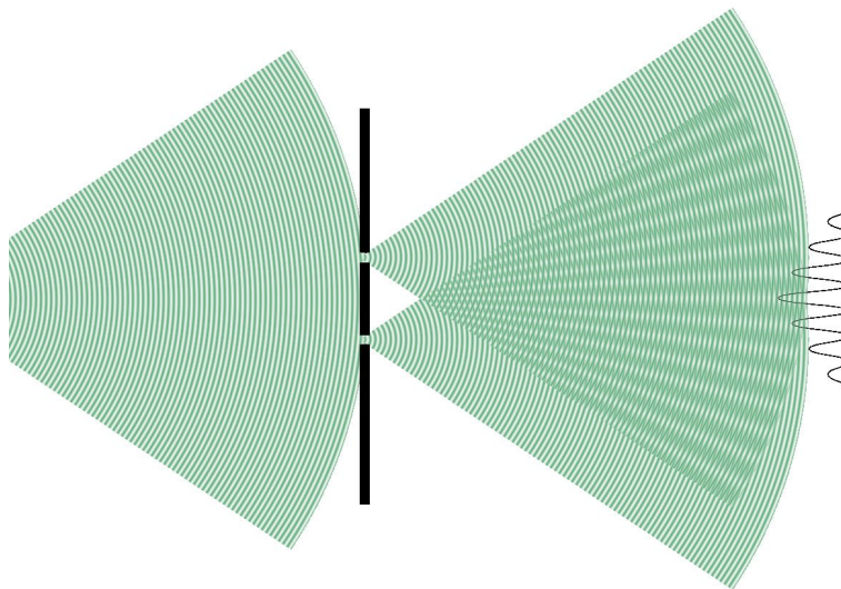
FIGURE 15 – Interprétation de l'expérience des fentes Young par les ondes.
