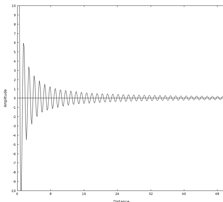
FIGURE 3 – Atténuation du son en fonction de la distance
