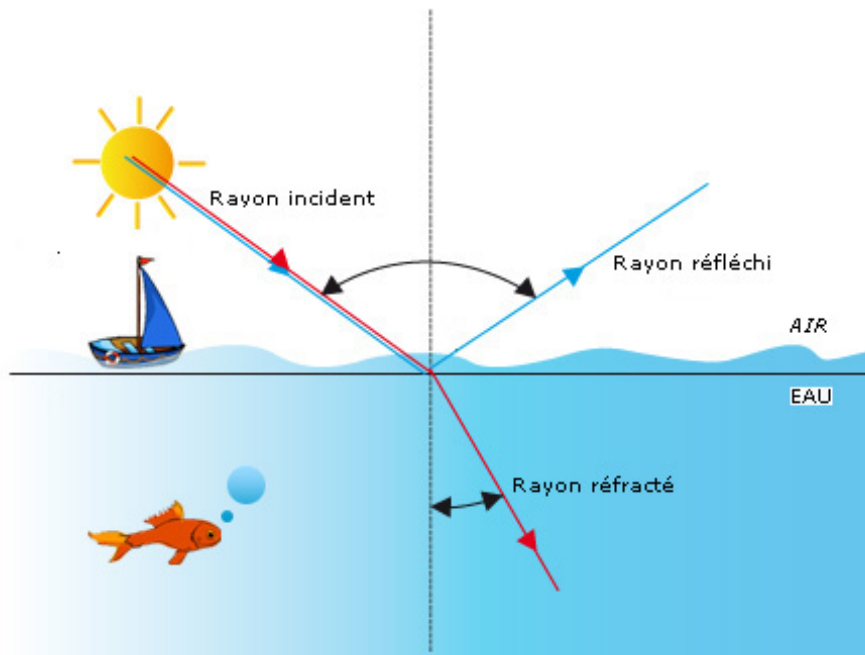
FIGURE 12 – Réflexion et réfraction de la lumière.
