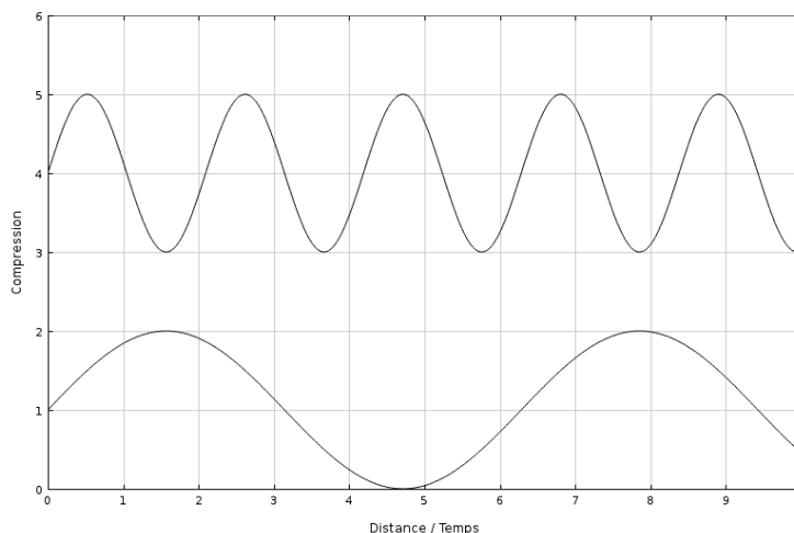
FIGURE 6 – L'onde du haut représente un son aigu. L'onde du bas représente un grave.
