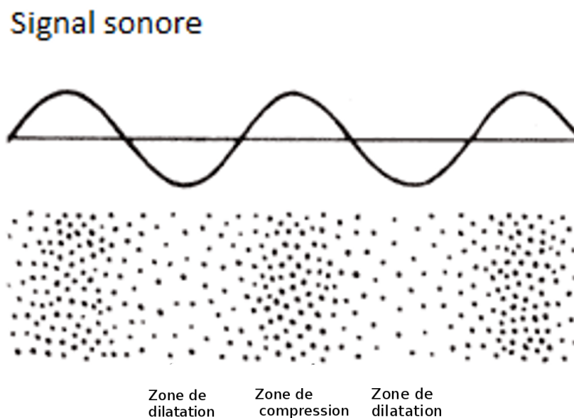
FIGURE 5 – Représentation d'une onde sonore
