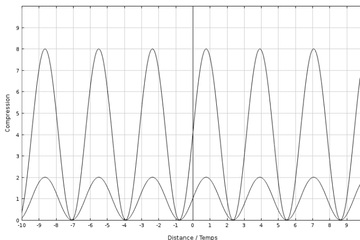
FIGURE 7 – Les deux ondes ont la même fréquence, mais celle qui a le plus de variation de compression a un volume plus important.
