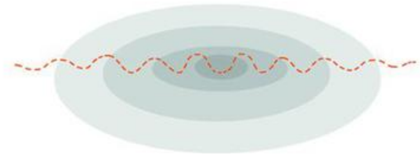
FIGURE 1 – Des ondes se formant sur un étang.
