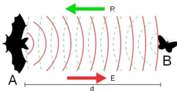
FIGURE 10 – La chauve-souris peut détecter les papillons en détectant les ondes qu'elle a émises et qui sont réfléchies par le papillon.
