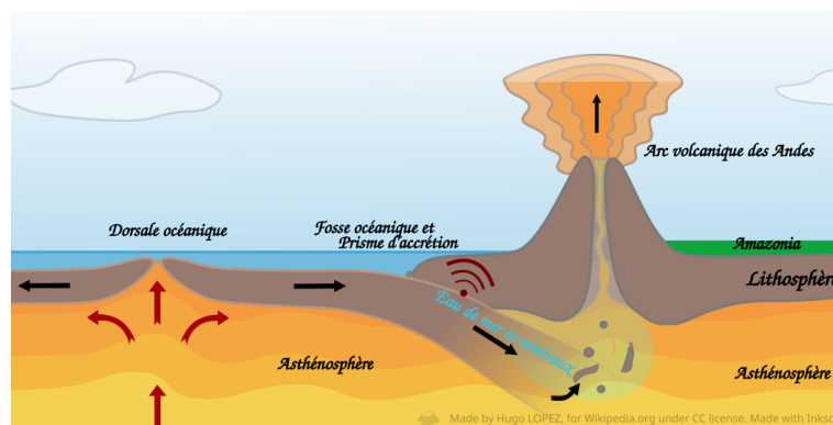
FIGURE 12 – Dynamique de la croûte terrestre (en exemple la plaque Nazca en face de la cote occidentale d'Amérique du Sud).
