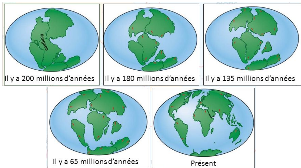
FIGURE 13 – Évolution des plaques tectoniques depuis 200 millions d'années
