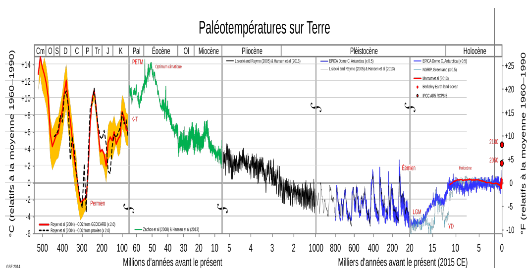
FIGURE 9 – Évolution de la température moyenne de la Terre (à partir de -500 millions d'années).
