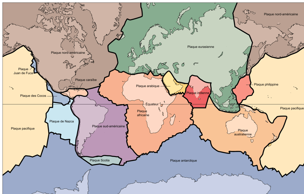
FIGURE 14 – Plaques tectoniques actuelles
