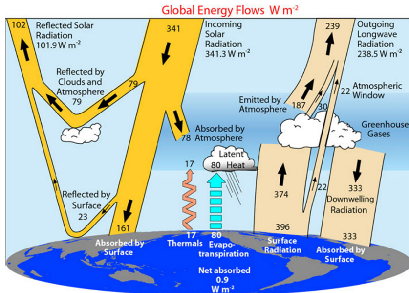
FIGURE 10 – Bilan radiatif de la Terre et effet de serre
