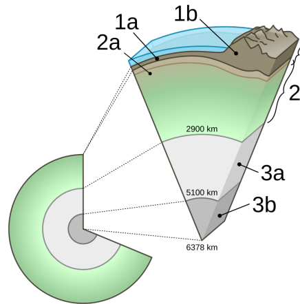
FIGURE 11 – Structure interne de la Terre
