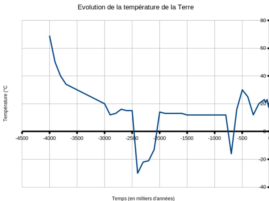
FIGURE 8 – Évolution de la température moyenne de la Terre (à partir de -3 milliards d'années).
