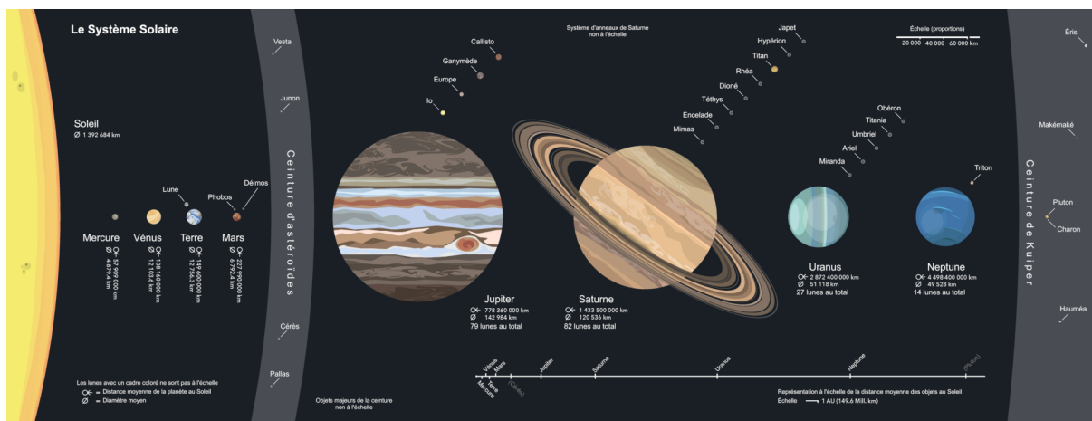
FIGURE 1 – Système solaire
