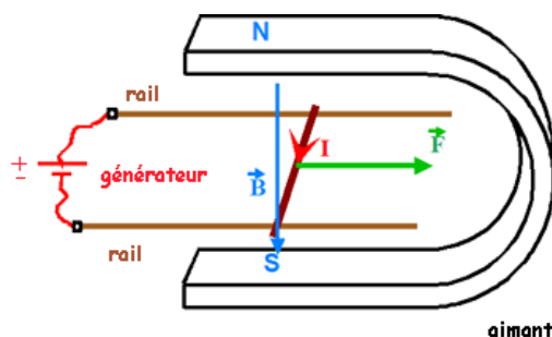
FIGURE 1 – Force induite par un courant continu et un aimant.
