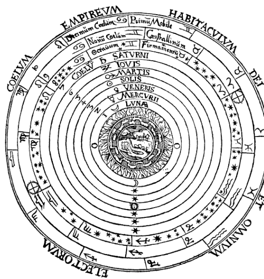
FIGURE 3 – Le monde selon Ptolémée.
