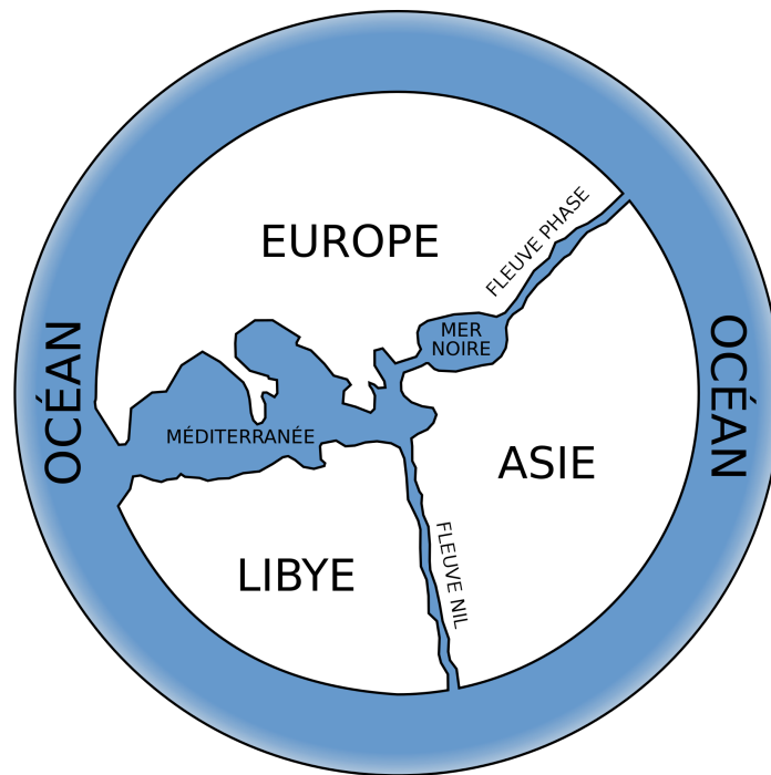
FIGURE 1 – Le monde d'Anaximandre
