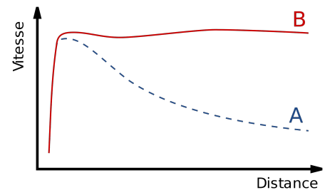
FIGURE 7 – Vitesse des objets par rapport à la distance du centre de la galaxie (A Théorie de Newton, B Données observées)
