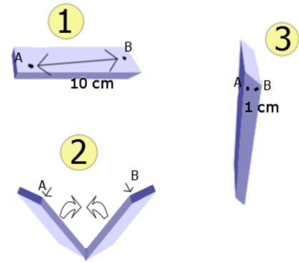
FIGURE 9 – Principe d'un trou de ver.
