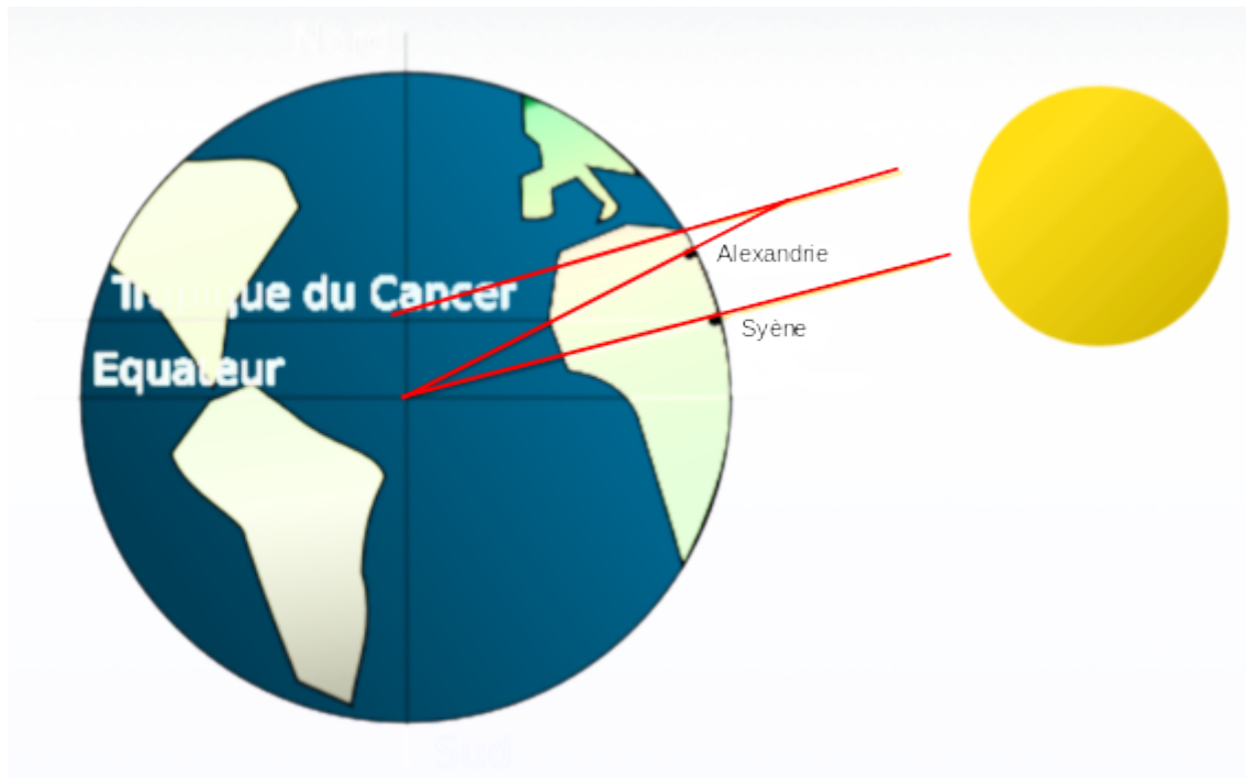
FIGURE 2 – Mesure de la circonférence de la Terre par Ératosthène
