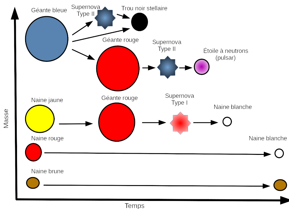
FIGURE 6 – Évolution des objets stellaires en fonction de la masse initiale.
