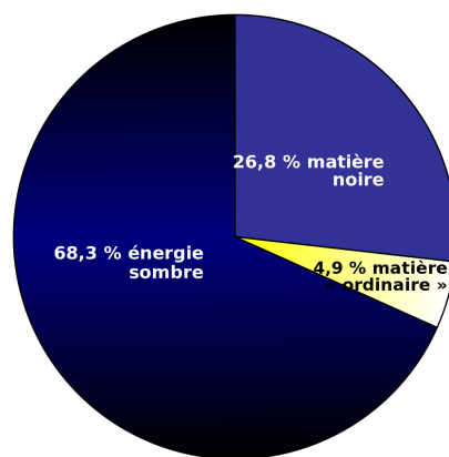
FIGURE 8 – Répartition de la matière de l'Univers
