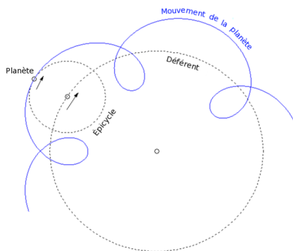
FIGURE 4 – Le mouvement des épicycles.
