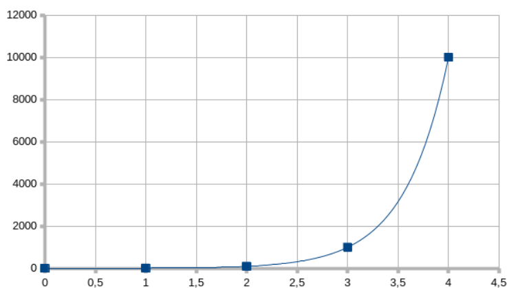
FIGURE 5 – Représentation graphique de f(x) = 10^x .
