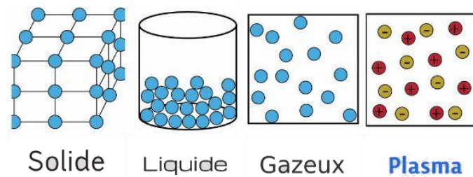
FIGURE 1 – Les 4 états de la matière.
